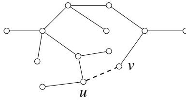
Figure 1: Wanneer in een boom T een lijn e = (u, v) wordt toegevoegd ontstaat een cykel. We kunnen e toevoegen en vervangen door elke lijn op die cykel en houden weer een boom over. Indien T een MST is, moet dus het gewicht van e groter zijn dan dat van elke andere lijn op de cykel.
